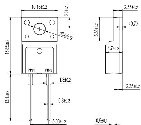
ITO-220AC HER8XXF
